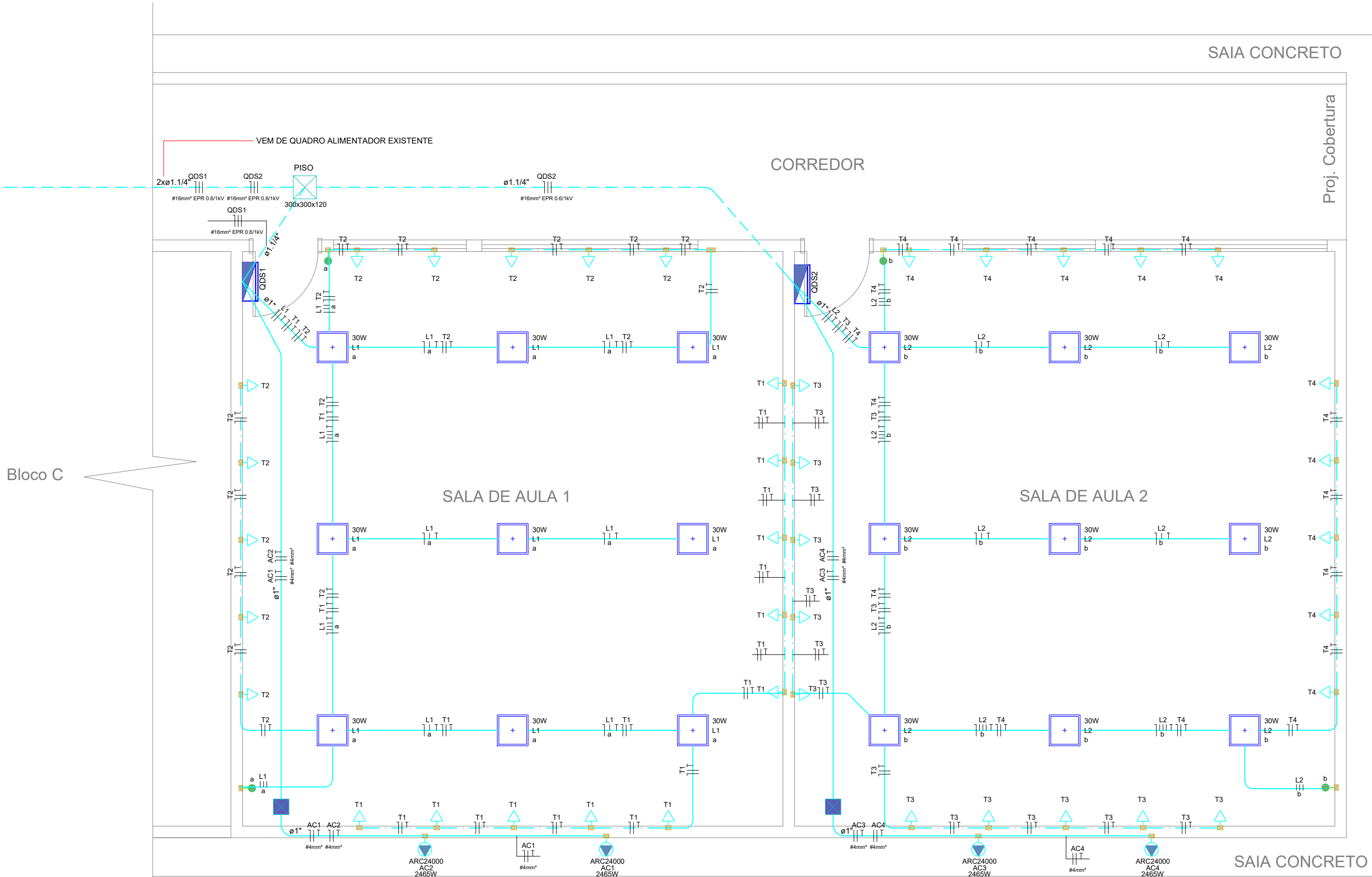
ENERGIA COMUM - SALAS 1:50
