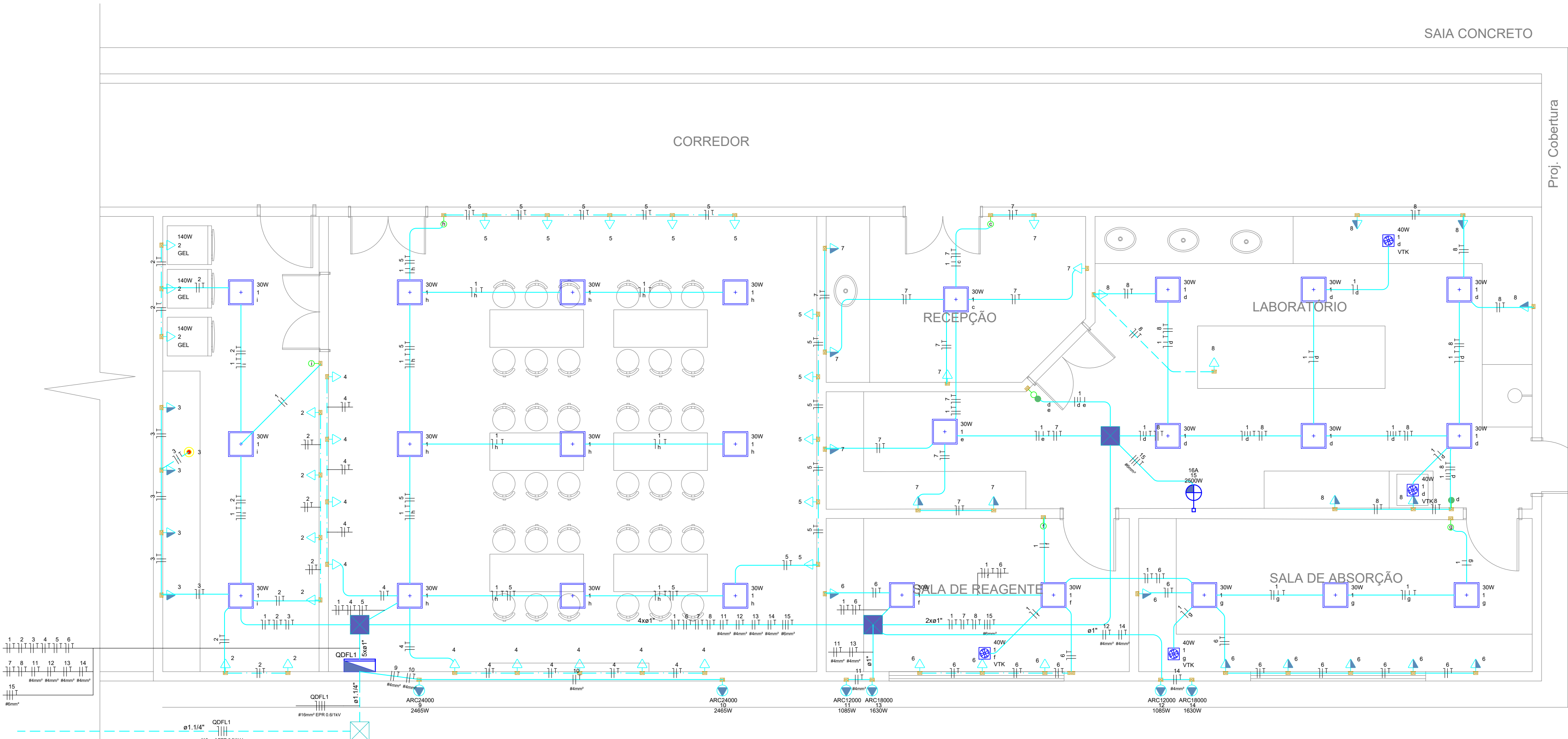
ENERGIA COMUM - BLOCO 1:50
