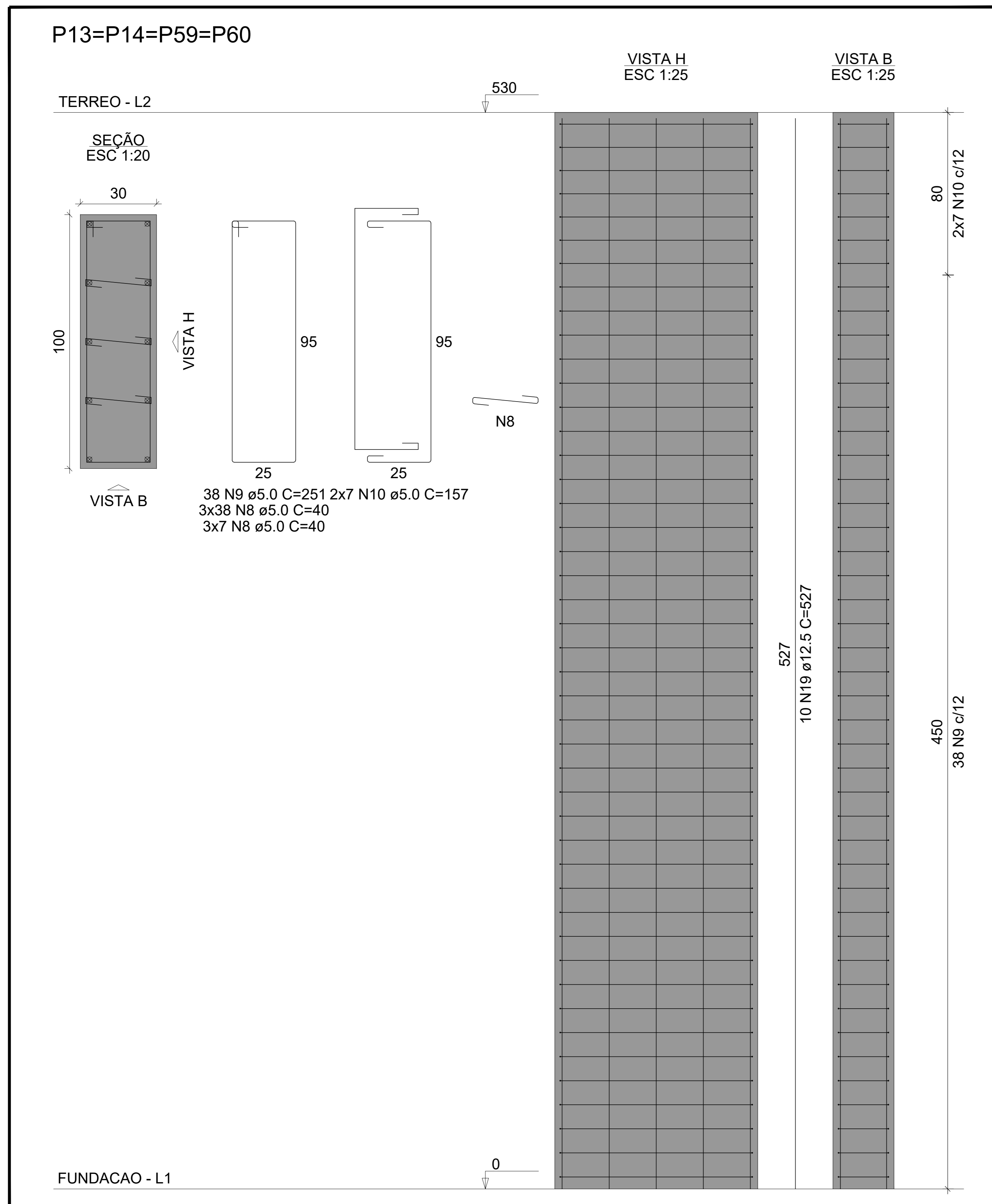
18.00 ARMADURAS - PILARES - TÉRREO ESCALA 1/E
