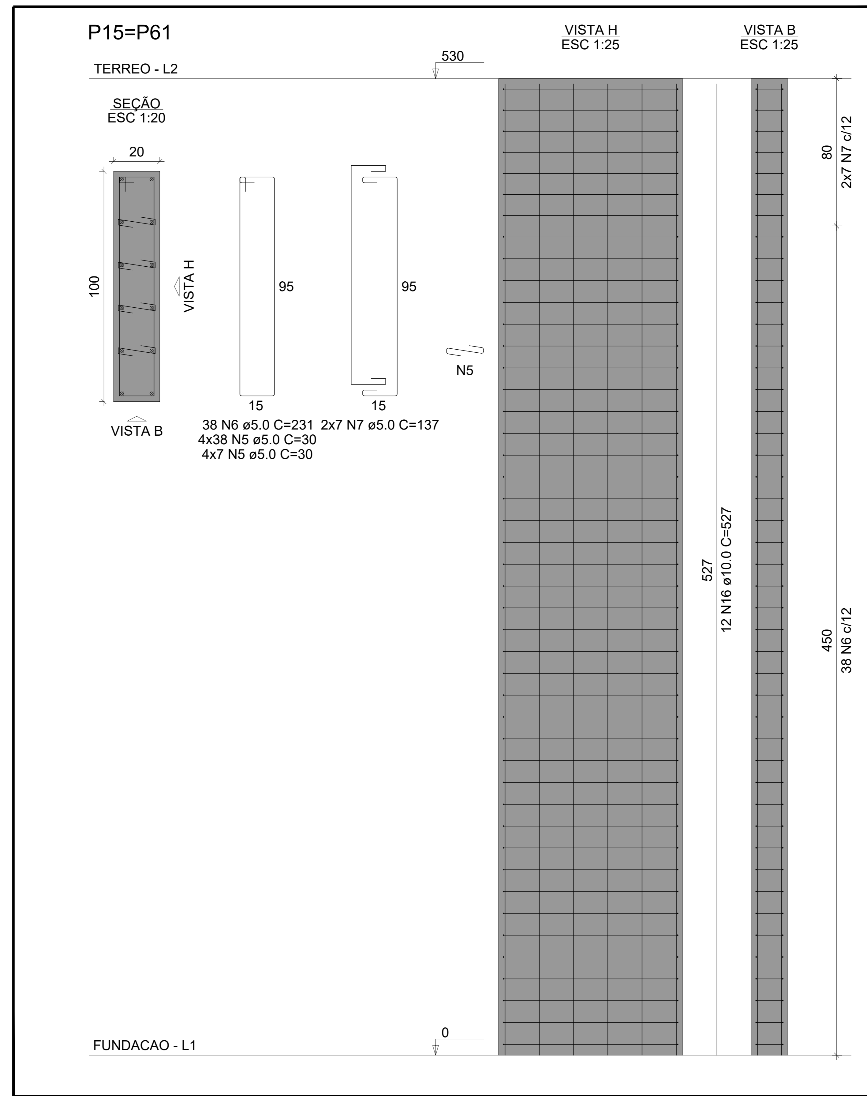
18.01 ARMADURAS - PILARES - TÉRREO ESCALA 1/E
