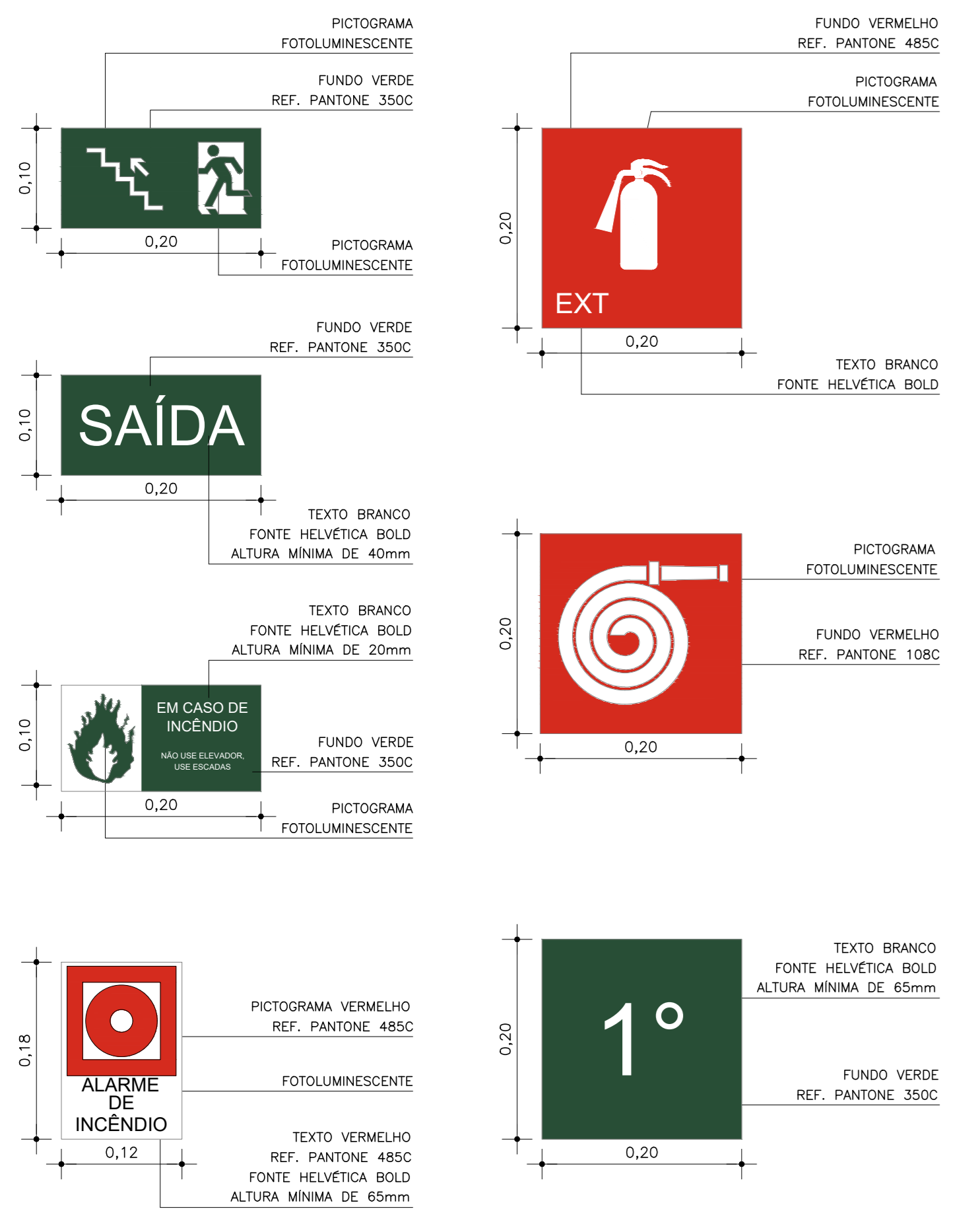
03.01 DETALHE - PLACA DE SINALIZAÇÃO ESCALA 1/E
