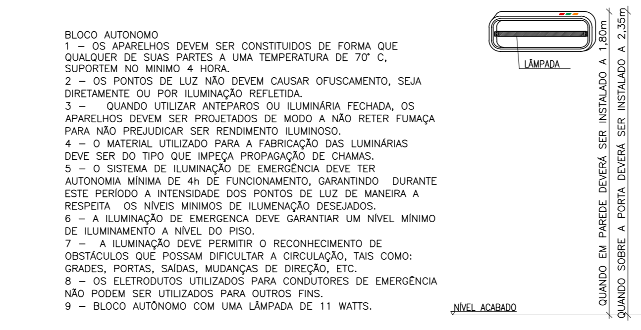
03.03 DETALHE - LUMINARIA DE EMERGÊNCIA ESCALA 1/E
