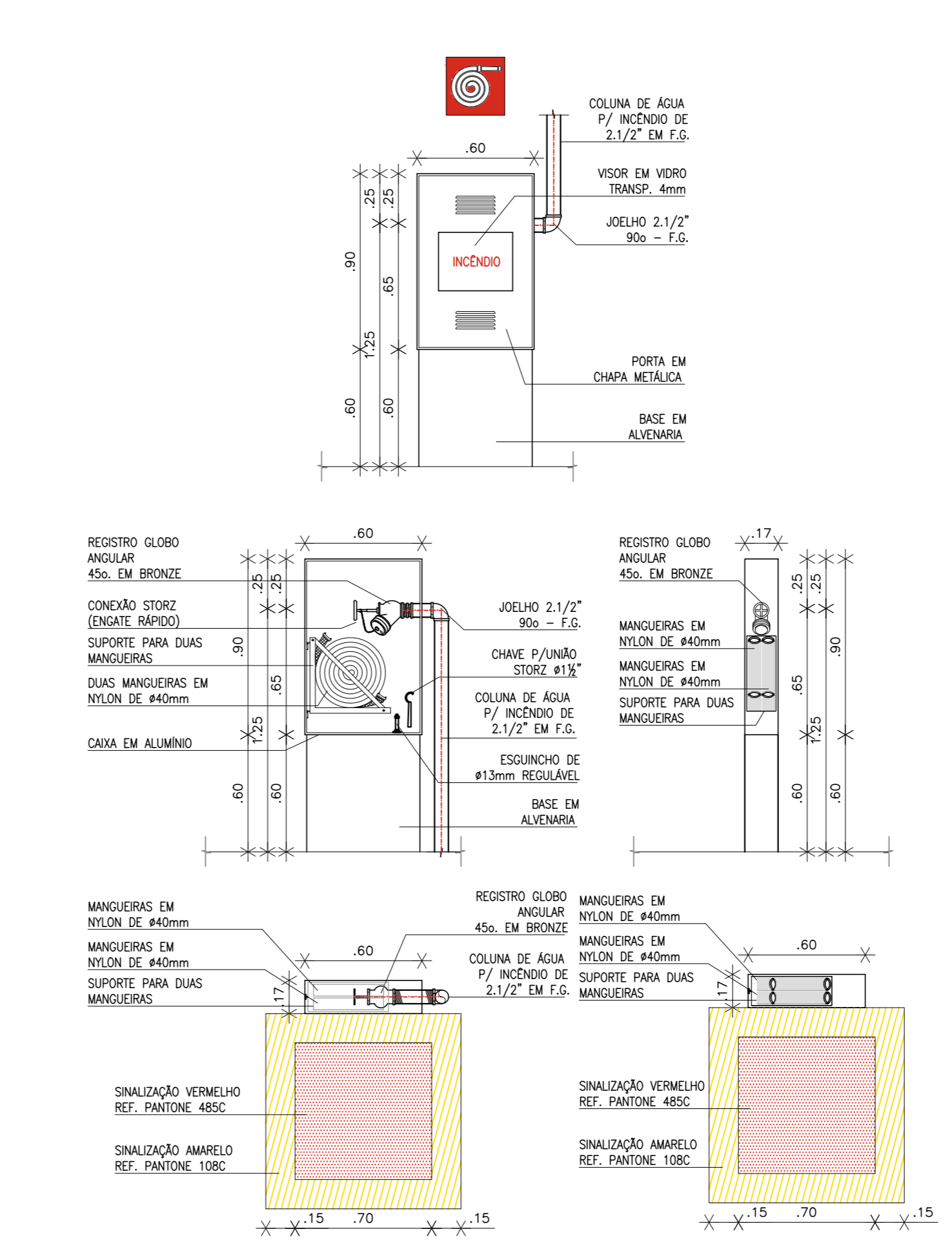
03.05 DETALHE - HIDRANTE ESCALA 1/E
