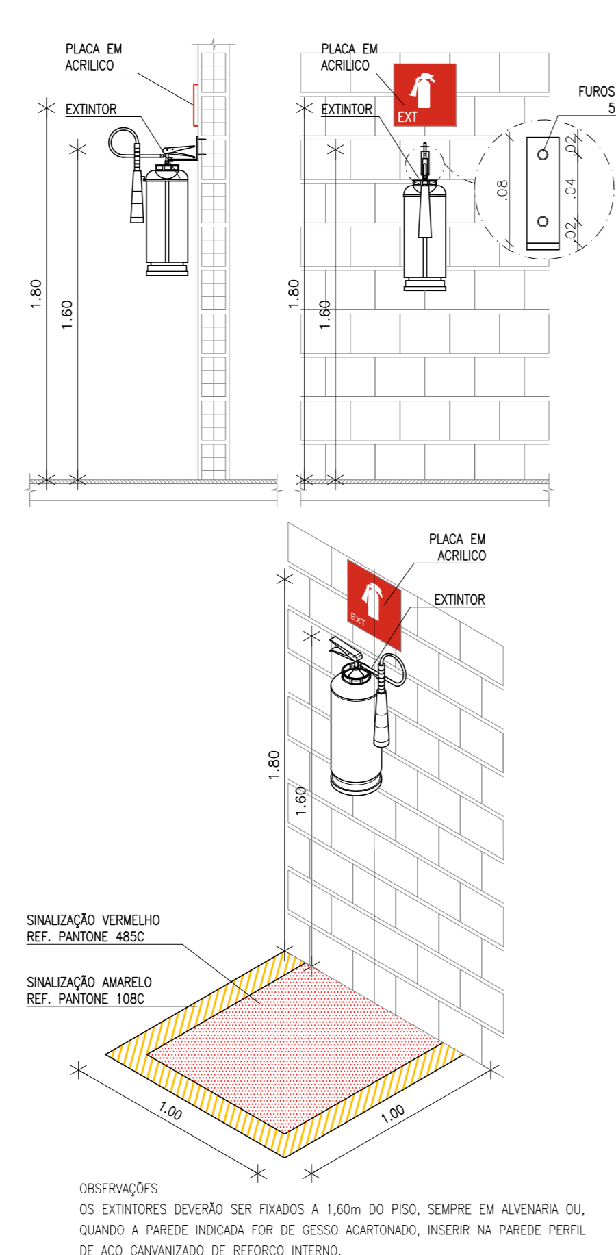
03.02 DETALHE - EXTINTOR ESCALA 1/E
