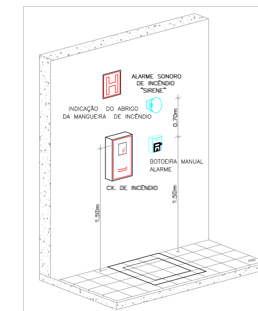
03.06 DETALHE - INSTALAÇÃO HID. E ALARME ESCALA 1/E
