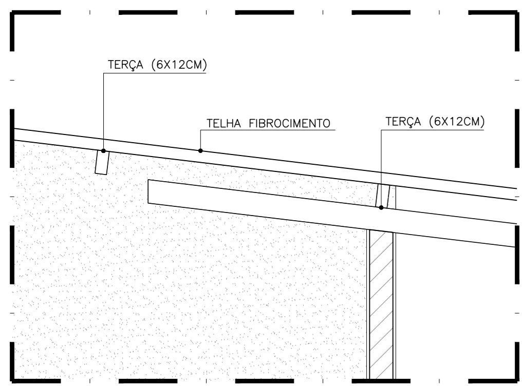
03.02 DETALHE 02 - TERÇA ESCALA 1/20
