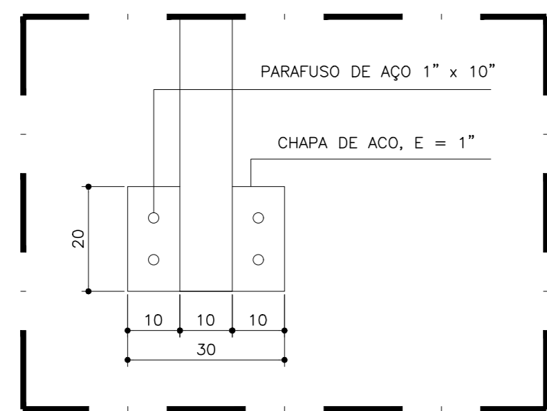
03.03 DETALHE 03 - LIGAÇÃO ESCALA 1/10
